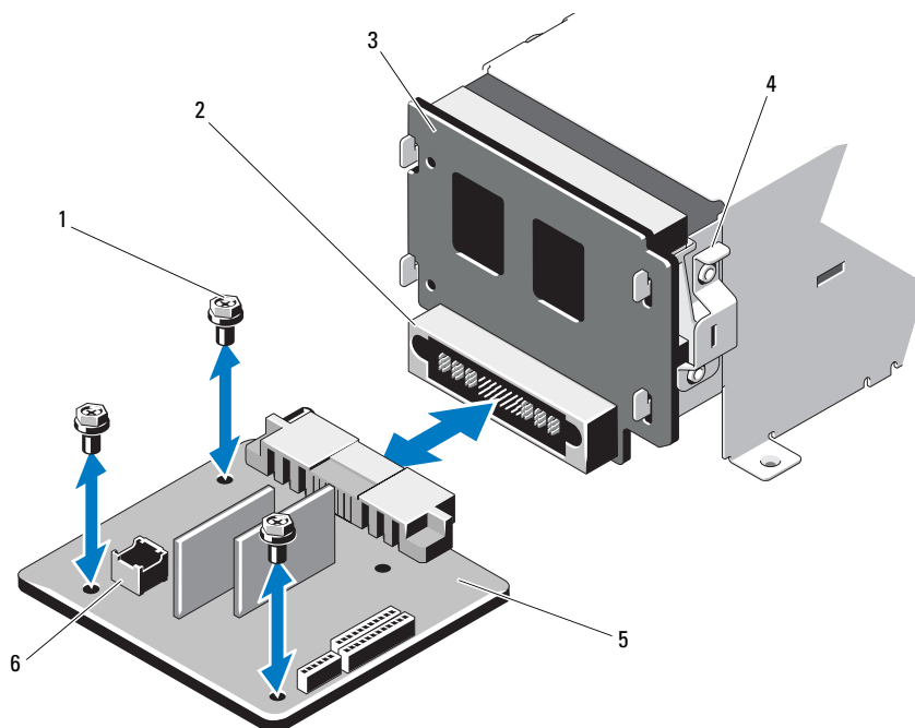
図 3-36 配電基板の取り外しと取り付け（ハードドライブ 12 台のシステム）
