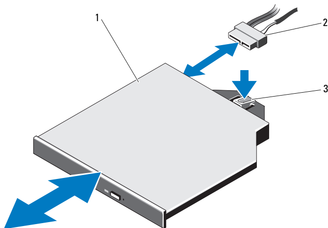
図 3-14 オプティカルドライブの取り外し
