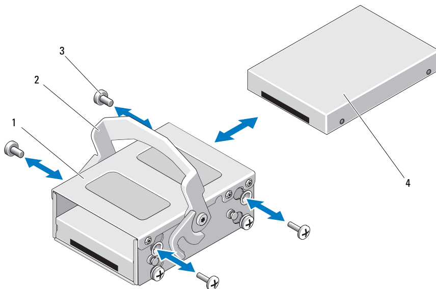
図 3-13 内蔵ハードドライブの内蔵ハードドライブベイへの取り付けと取り外し
