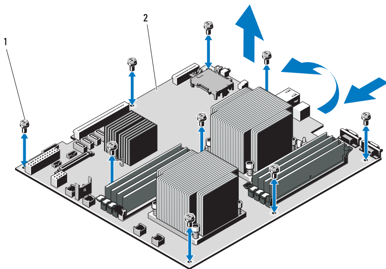
図 3-37 システム基板の取り外しと取り付け
