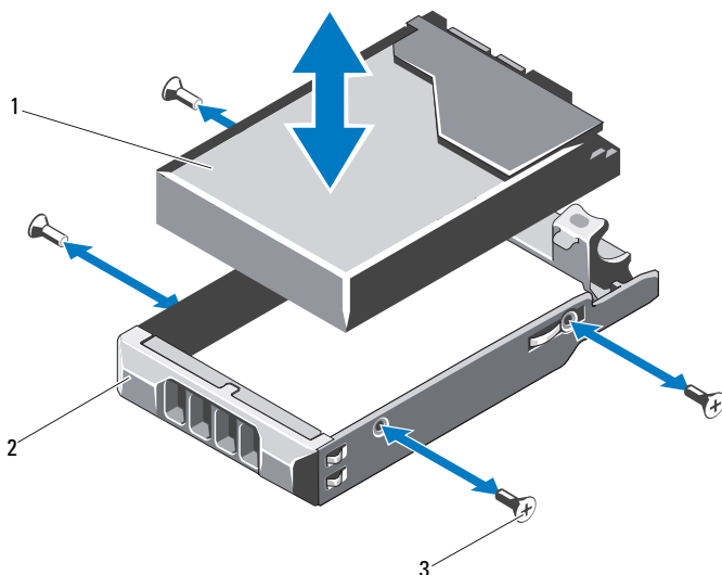
図 3-11 ケーブル接続式ハードドライブをハードドライブキャリアに取り付ける方法
