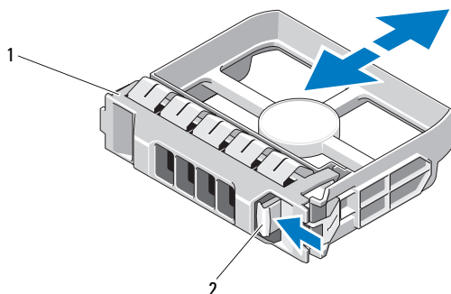
図 3-7 ハードドライブダミーの取り外しまたは取り付け
