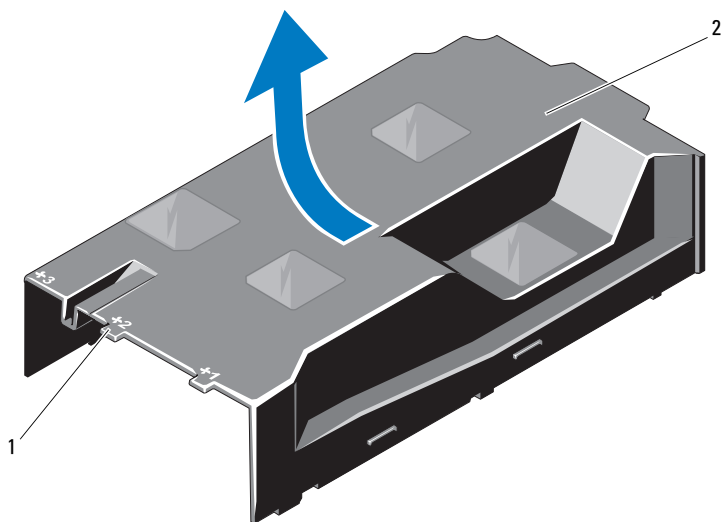
図 3-6 冷却用エアフローカバーの取り付けと取り外し
