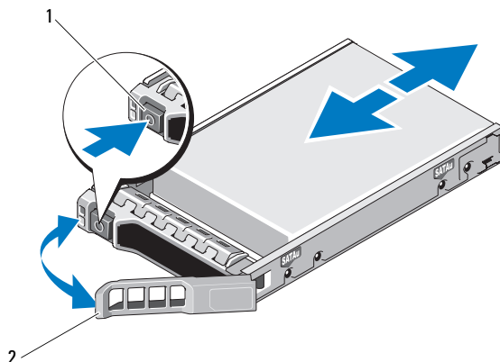
図 3-8 ホットスワップ対応ハードドライブの取り外しと取り付け
