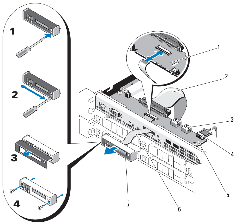
図 3-32 コントロールパネル—LCD の取り外しと取り付け
