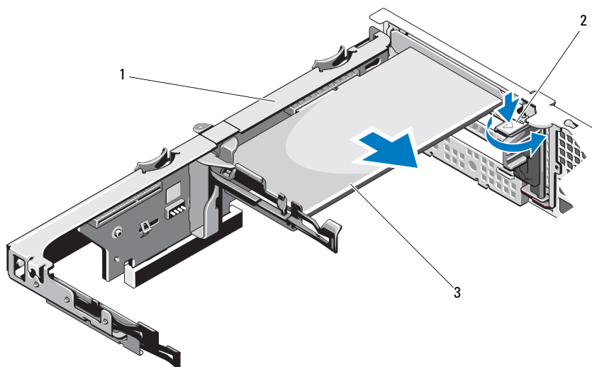
図 3-20 拡張カードの取り付けまたは取り外し
