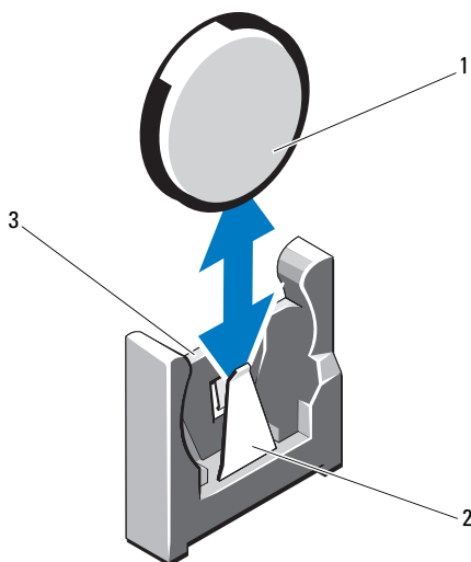
図 3-28 システムバッテリーの交換
