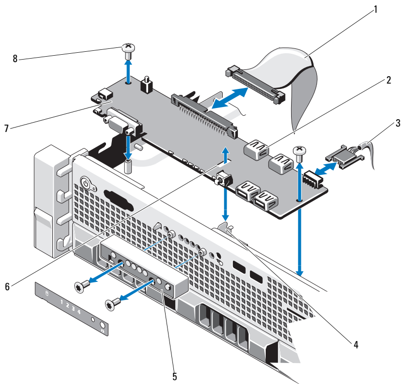
図 3-30 コントロールパネル—LED の取り外しと取り付け (ハードドライブ 4 台のシステム)
