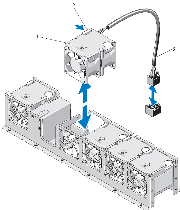
図 3-16 ファンを取り外しと取り付け (ハードドライブ 12 台のシステム)
