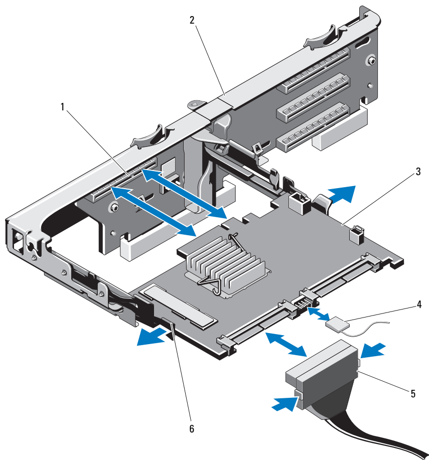
図 3-22 ストレージコントローラカードの取り付けと取り外し
