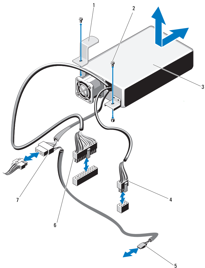
図 3-18 非冗長電源ユニットの取り外しと取り付け
