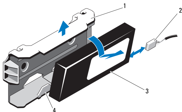
図 3-29 RAID バッテリーの取り付けと取り外し
