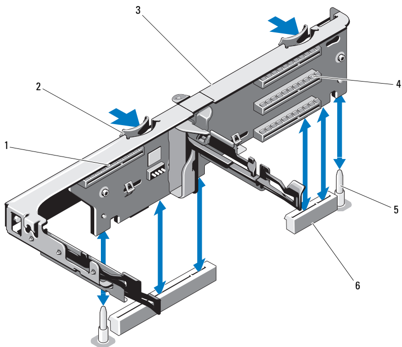
図 3-21 拡張カードライザーの取り付けまたは取り外し
