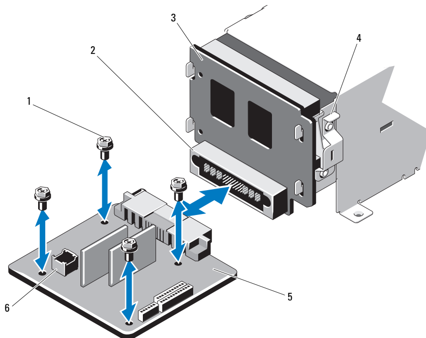
図 3-35 配電基板の取り外しと取り付け（ハードドライブ 8 台のシステム）
