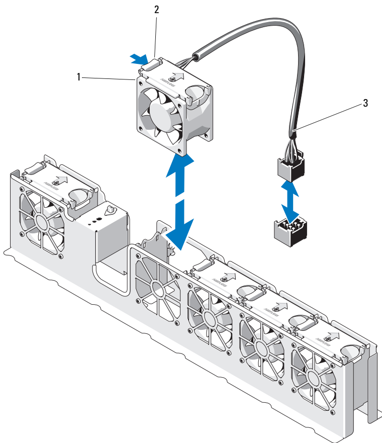
図 3-15 ファンを取り外しと取り付け (ハードドライブ 8 台のシステム)
