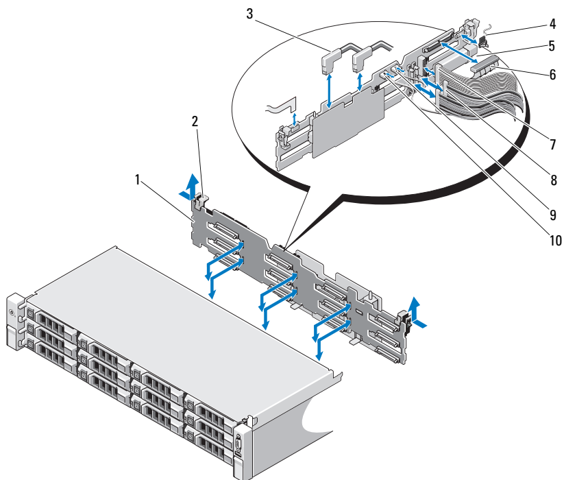
図 3-34 SAS バックプレーンの取り外しと取り付け（ハードドライブ 12 台のシステム）
