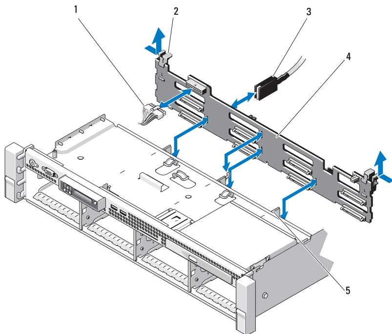
図 3-33 SAS バックプレーンの取り外しと取り付け (ハードドライブ 8 台のシステム)
