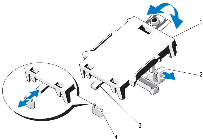
図 3-23 iDRAC6 Express カードの取り付けまたは取り外し
