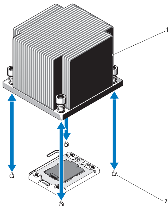
図 3-26 ヒートシンクの取り付けと取り外し
