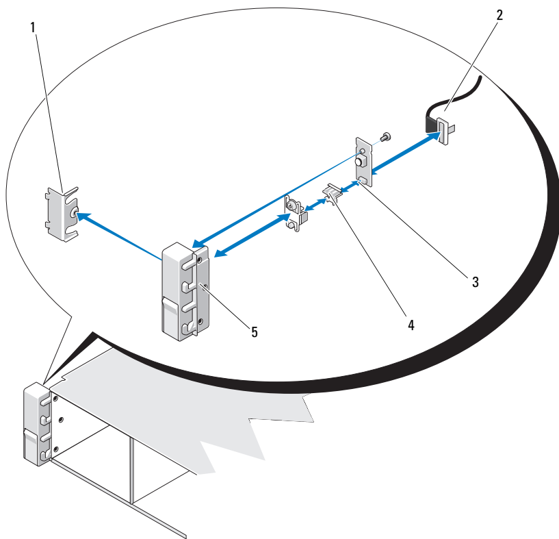
図 3-31 コントロールパネル —LED の取り外しと取り付け（ハードドライブ 12 台のシステム）
