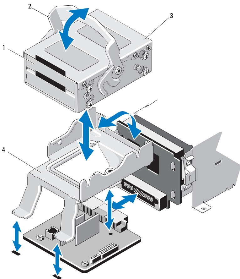
図 3-12 内蔵ハードドライブベイの取り付けと取り外し
