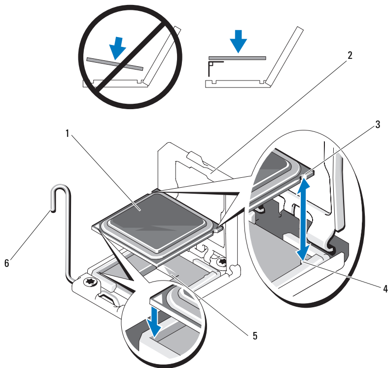
図 3-27 プロセッサの取り付けと取り外し
